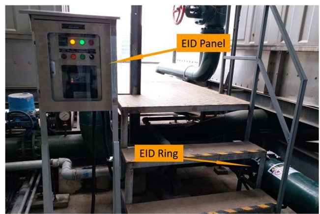
修頓中心水冷式製冷機加裝電磁感應式防水垢裝置
